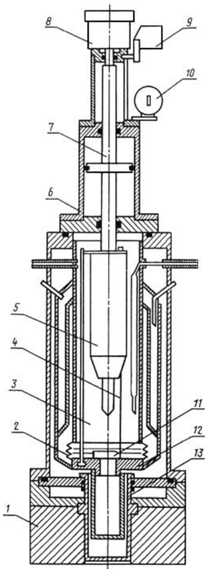
1 - основание копра; 2 - сильфон; 3 - объем для заливки жидкого хладагента; 4 - тяги; 5 - молот; 6 - пневмоцилиндр; 7 - шток; 8 - шариковый замок; 9 - шторка; 10 - фотодатчик; 11 - образец; 12 - наковальня; 13 - динамометр
