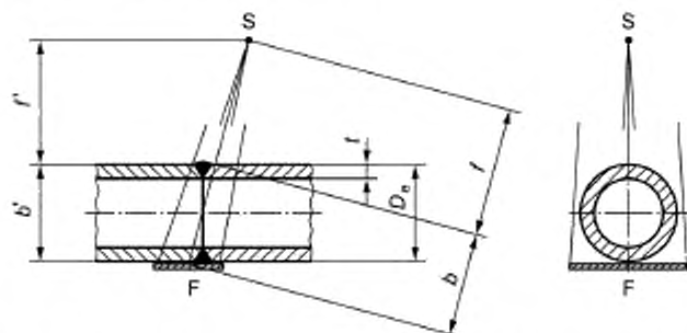
Рисунок 11 — Схема контроля изогнутых объектов для контроля двух стенок при просвечивании через две стенки (двойное изображение, источник излучения и пленка — снаружи)
