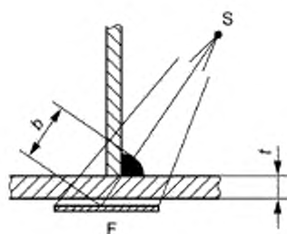
а) Схема контроля без кромочного компенсатора
