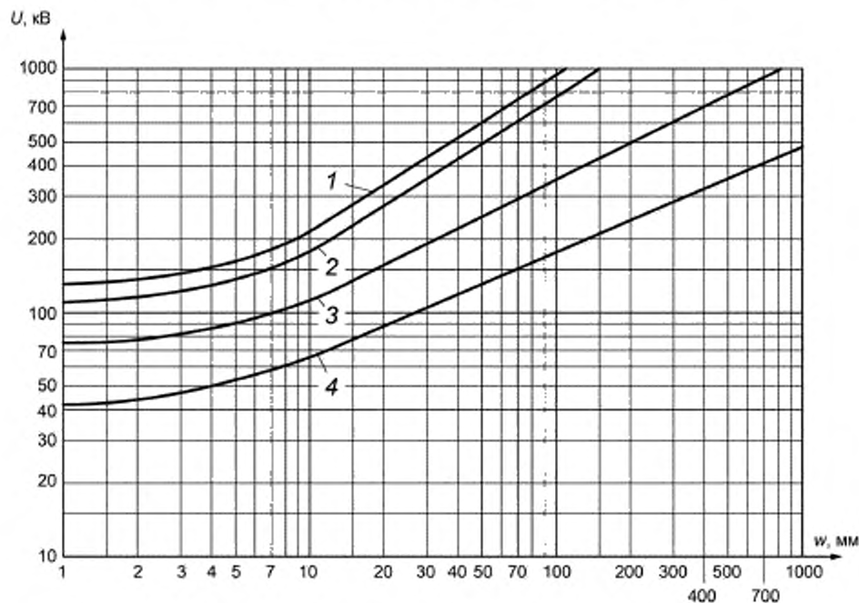
Рисунок 20 — Максимальное напряжение на рентгеновской трубке для источников с максимальным возможным напряжением до 1000 кВ как функция от просвечиваемой толщины и материала
