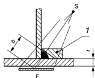
б) Схема контроля с кромочным компенсатором
