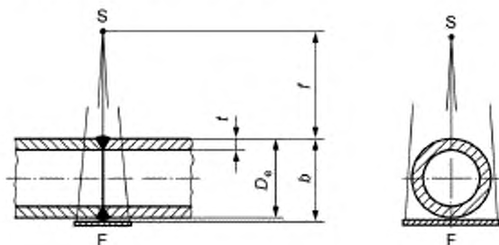
Рисунок 12 — Схема контроля изогнутых объектов для контроля двух стенок при просвечивании через две стенки (двойное изображение, источник излучения и пленка — снаружи)
