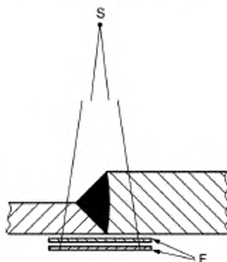
Рисунок 19 — Схема контроля с использованием нескольких пленок
