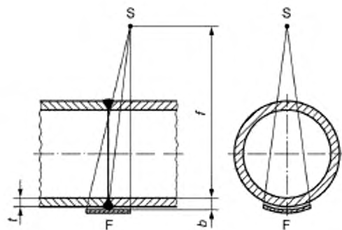
Рисунок 13 — Схема контроля изогнутых объектов при просвечивании через две стенки (одно изображение) для контроля стенки, ближайшей к пленке; IQI должен располагаться со стороны пленки
