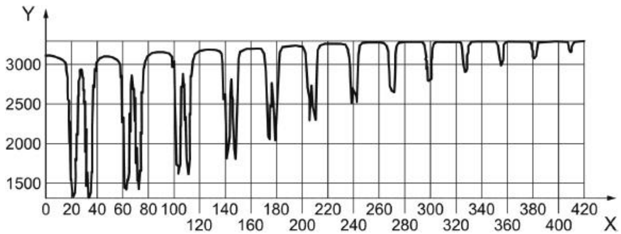
b - Профиль IQI двухпроводочного типа, усредненный, как минимум, по 21 линии
