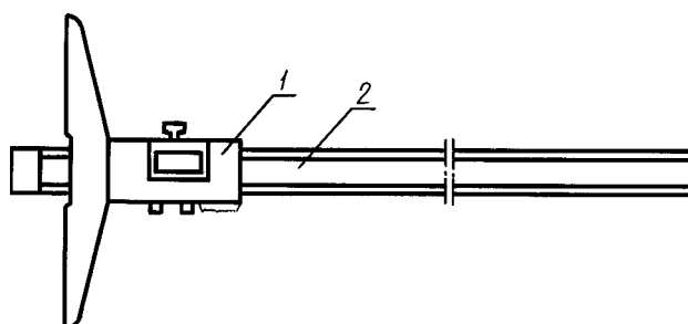
Тип ШГЦТ
