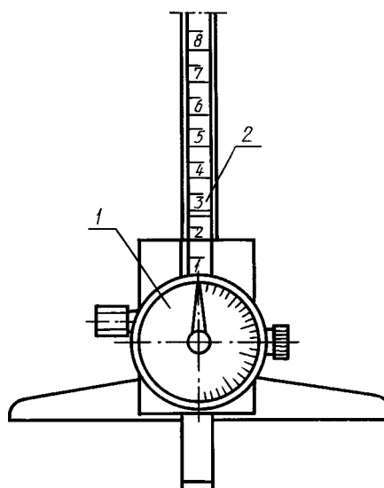
Тип ШГК
