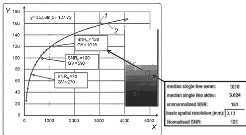
1 — измеренное значение на ступенчатом клине; 2 — кривая, аппроксимирующая результаты измерений на ступенчатом клине; X — значение градации серого GV; Y — нормализованное SNR N
