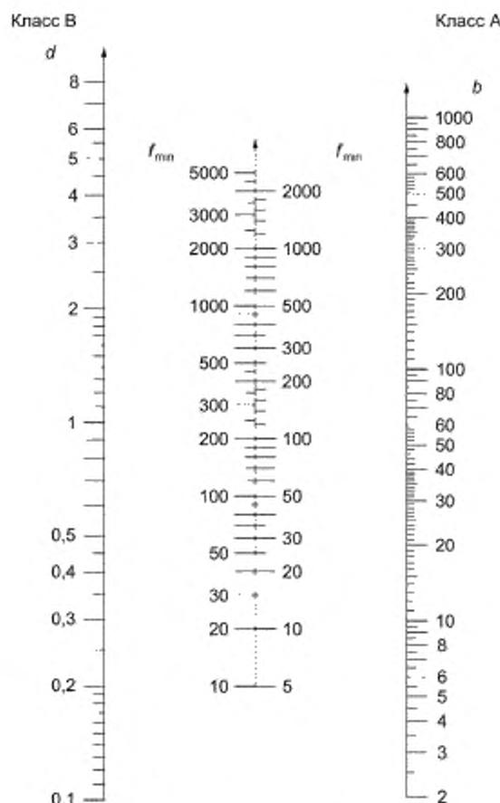
Рисунок 21 — Номограмма для определения минимального расстояния от источника излучения до объекта контроля f_{\min} в зависимости от расстояния от объекта контроля до детектора b и размера источника излучения d
