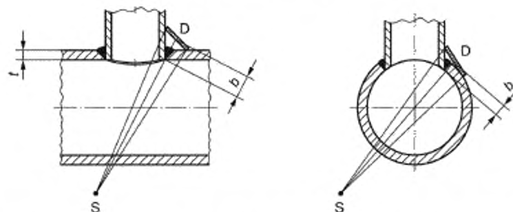
Рисунок 16 — Схема контроля изогнутых объектов при просвечивании через две стенки (одно изображение) для оценивания стенки, ближайшей к детектору
