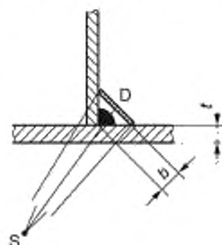
Рисунок 18 — Схема контроля при просвечивании угловых сварных швов
