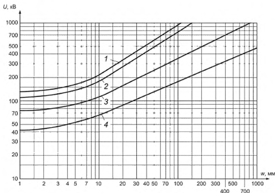
U — напряжение на рентгеновской трубке; w — просвечиваемая толщина; 1 — медь/никель и сплавы на их основе; 2 — сталь; 3 — титан и сплавы на его основе; 4 — алюминий и сплавы на его основе
