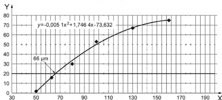
б — Интерполяция зависимости глубины модуляции от диаметра парных проволок (для определения SR_b ). Значение 20 % определяется из пересечения с линией 20 %, в результате чего iSR_b = 66 \text{ мкм}
