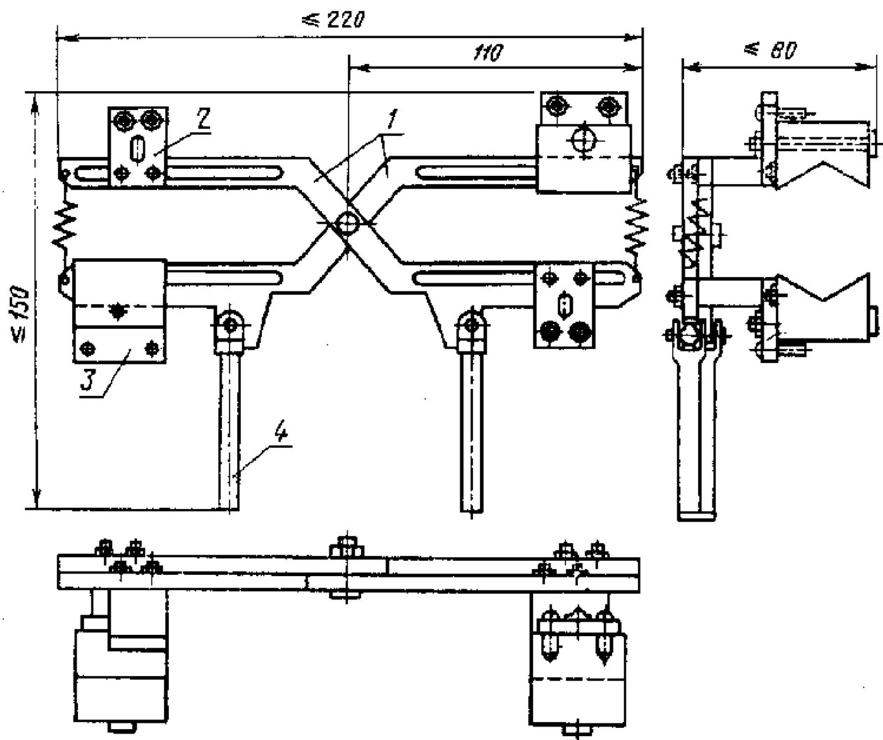
1 - рычаги; 2 - планка крепления искателя; 3 - фиксатор; 4 - рукоятка Черт. 1
