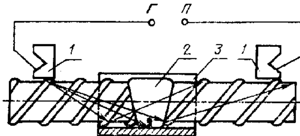
1 - наклонные искатели; 2 - сварное соединение; 3 - скоба-накладка; Г - выход к генератору ультразвуковых колебаний; П- вывод к приемнику Черт.2
