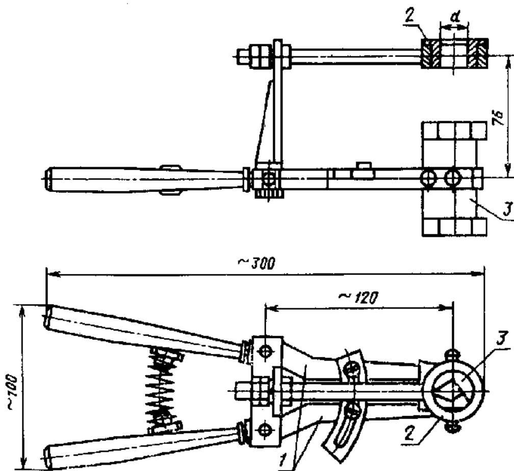
1 - рычаги; 2 - ограничительное кольцо; 3 - фиксатор Черт. 3
